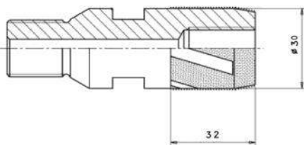
Body -Corpo
